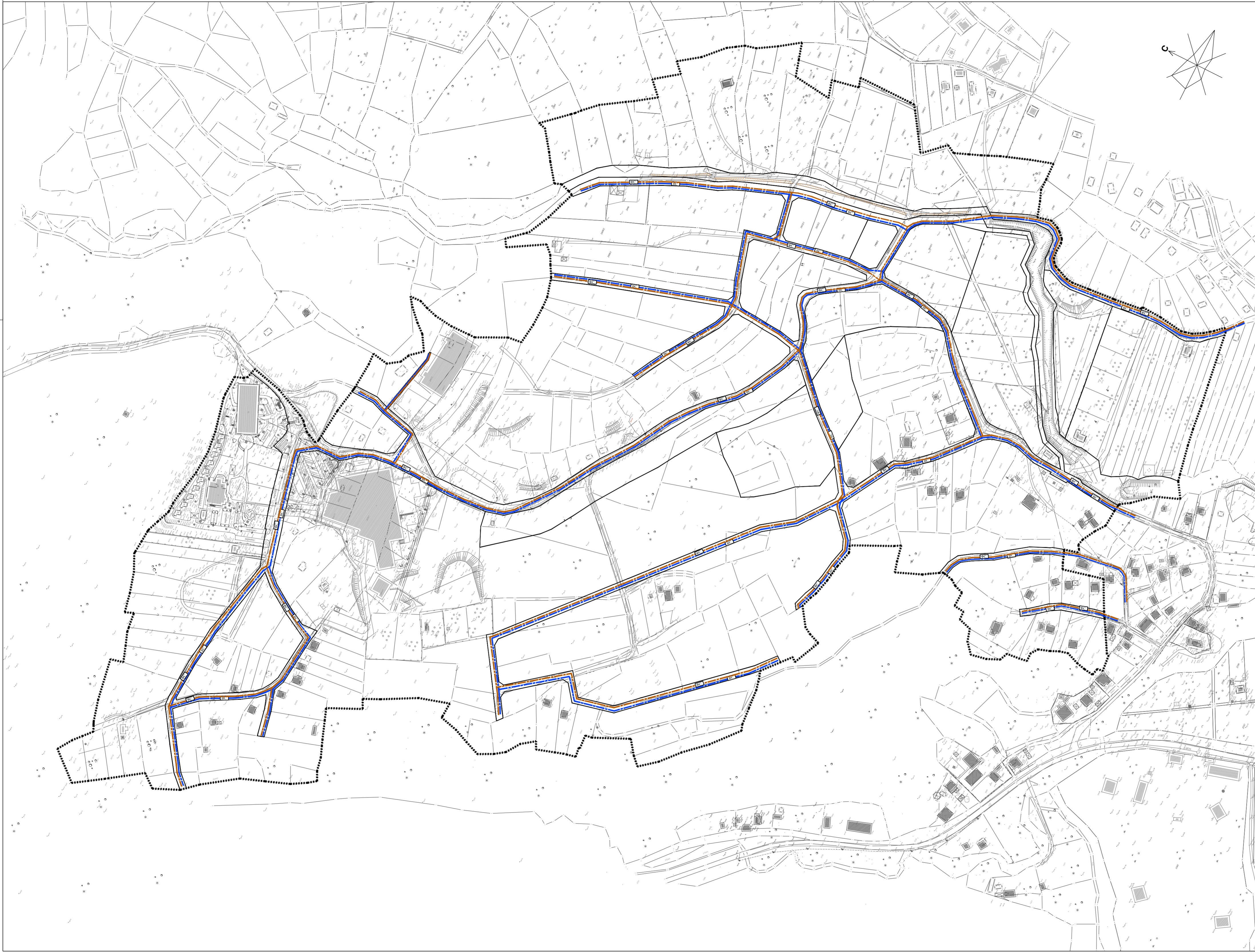
ПЛАН ВОДОВОДНЕ И КАНАЛИЗАЦИОНЕ ИНФРАСТРУКТУРЕ ЗА ПОДРУЧЈЕ ДЕТАЉНЕ РАЗРАДЕ
